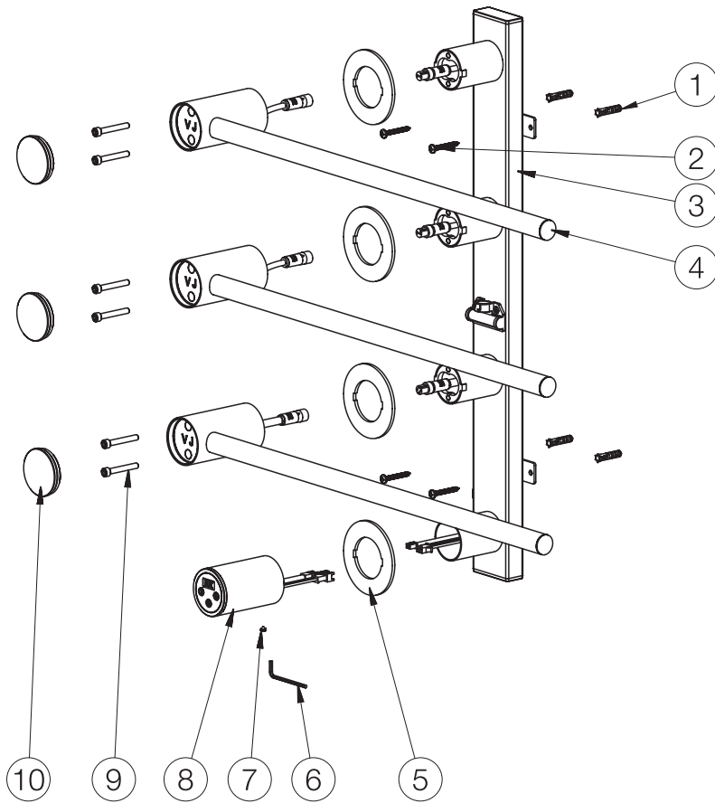
ТИПОВОЙ СОСТАВ КОМПЛЕКТА (НА ПРИМЕРЕ WW-AL313)
