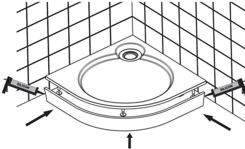
Рис.4. Обработка швов силиконом и установка экрана
