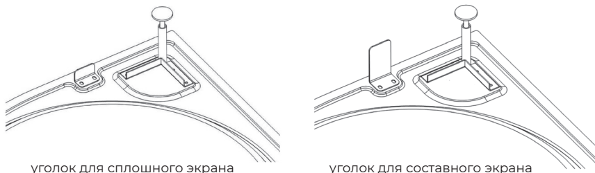
Рис.2. Виды монтажных уголков
